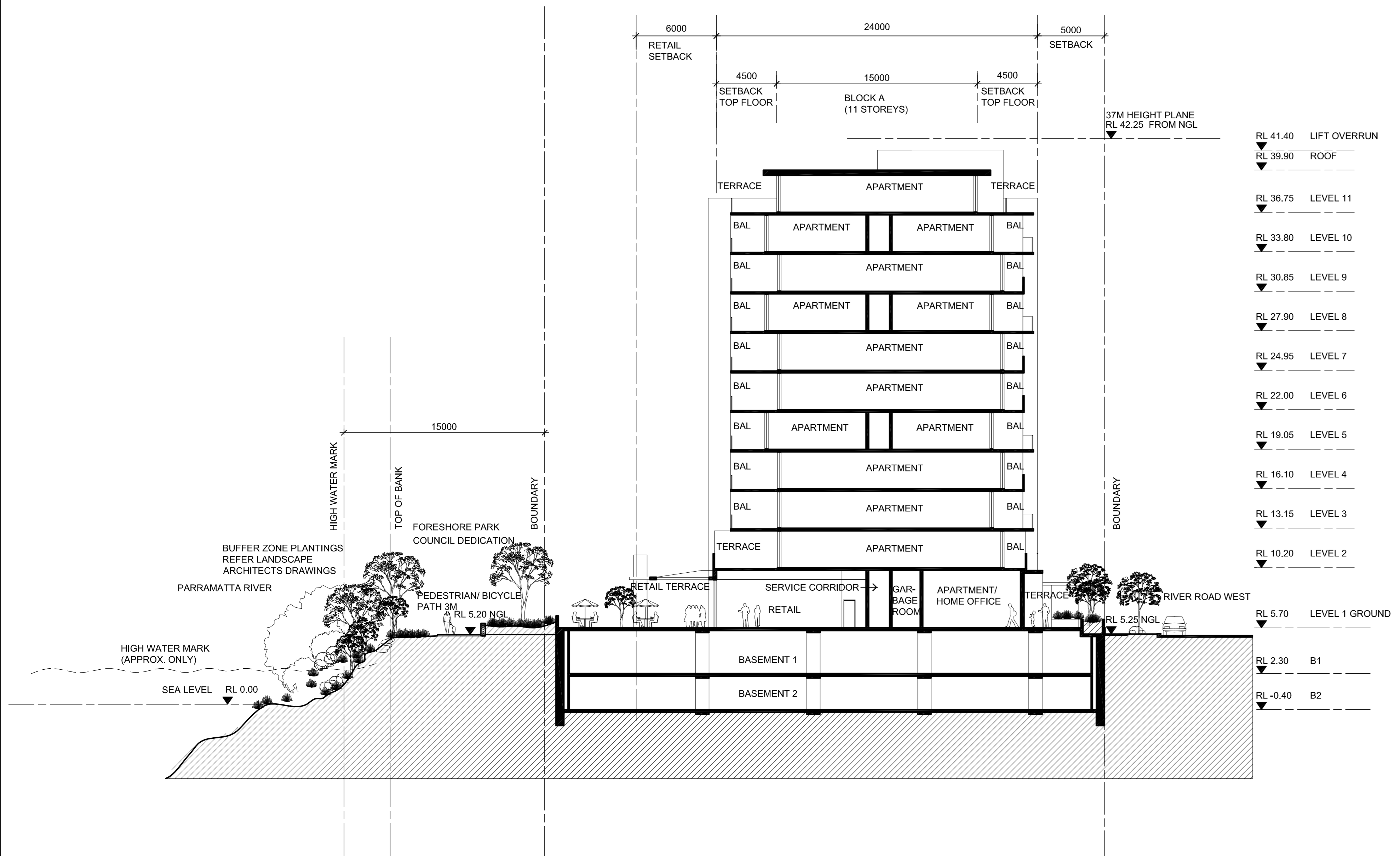
01 SECTION A-A
